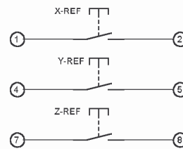
Verdrahtungsbeispiel mit mechanischen Schließern
