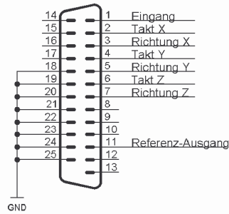
SIGNALEIN-/AUSGÄNGE 25-pol Stecker
